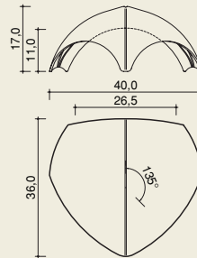
Walmkappe Universal III (dreiachsig)
