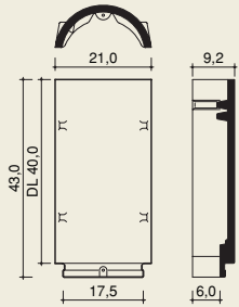
First Nr. 40 (2,5 Stück/m) bis 35° Neigung
