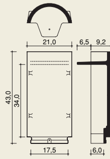
First-Anfang-Endziegel Nr. 40
