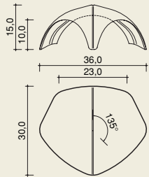
Walmkappe Universal I (dreiachsig)
