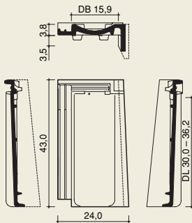
Ortgangziegel, rechts (3,0 Stück/m)
