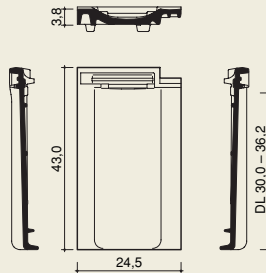
Doppelwulstziegel (3,0 Stück/m)
