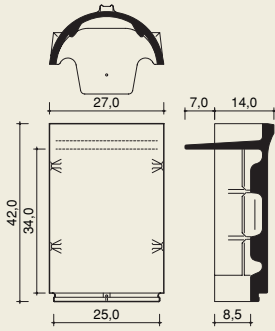
First-Anfang-Endziegel Nr. 60
